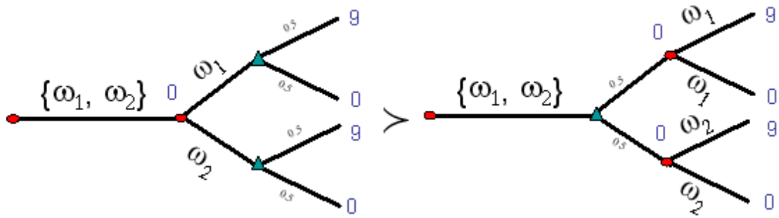
Fig. 9 k \succ k'
