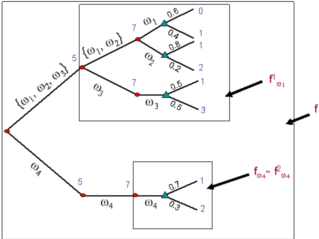
Fig. 2 f \in F_1^2
